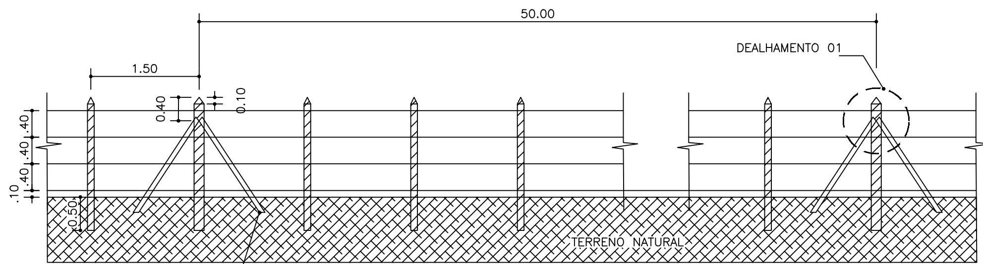
CORTE A ESCALA 1:75
