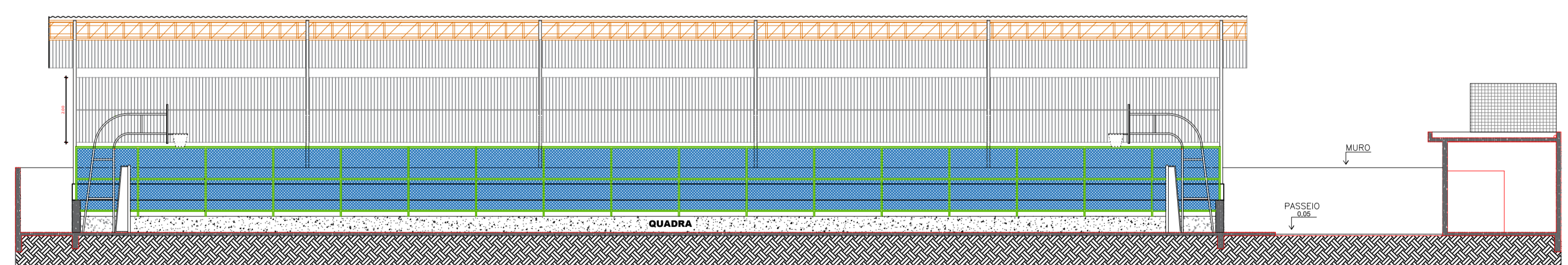
CORTE CC ESCALA 1:125
