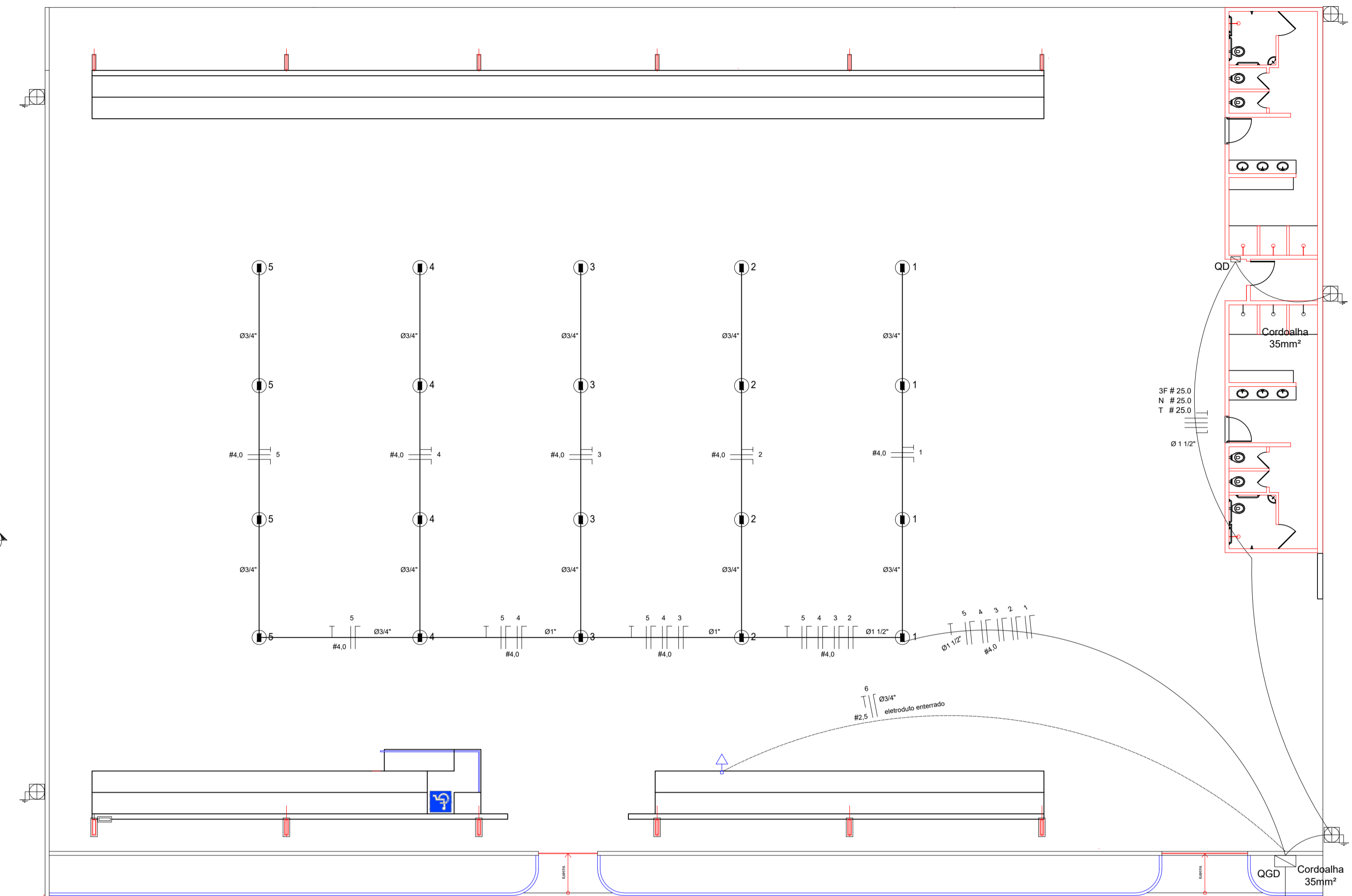
PLANTA BAIXA ELÉTRICA ESCALA 1:125
