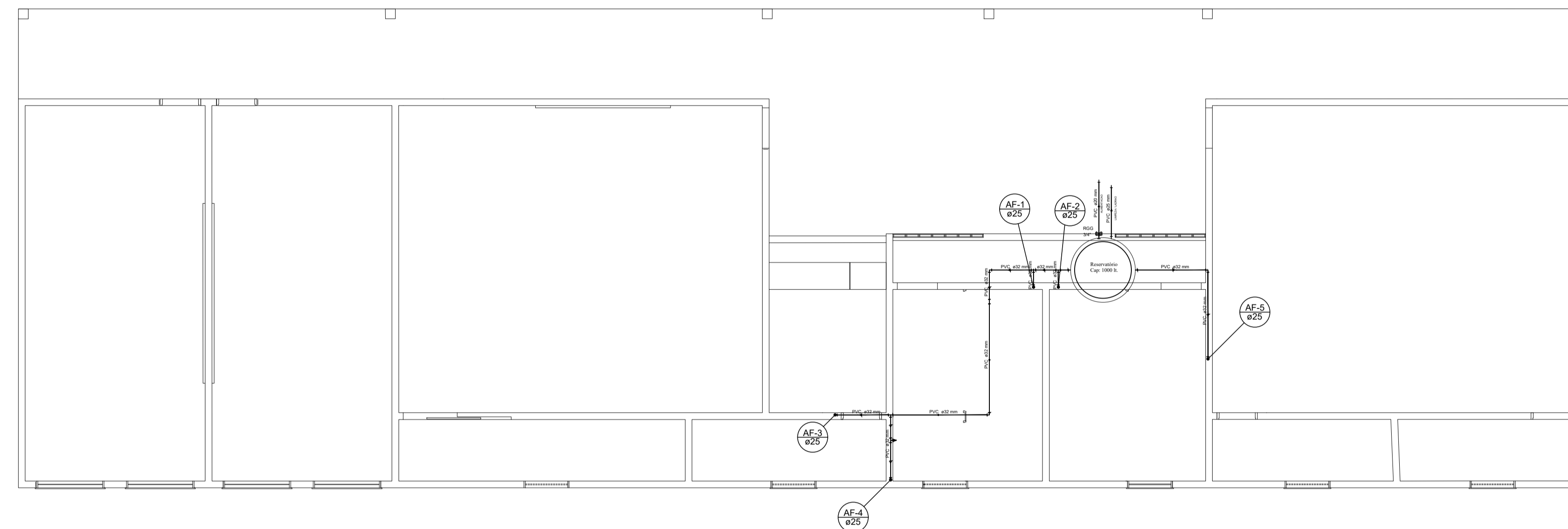
PLANTA BAIXA CAIXA D'ÁGUA escala 1:75
