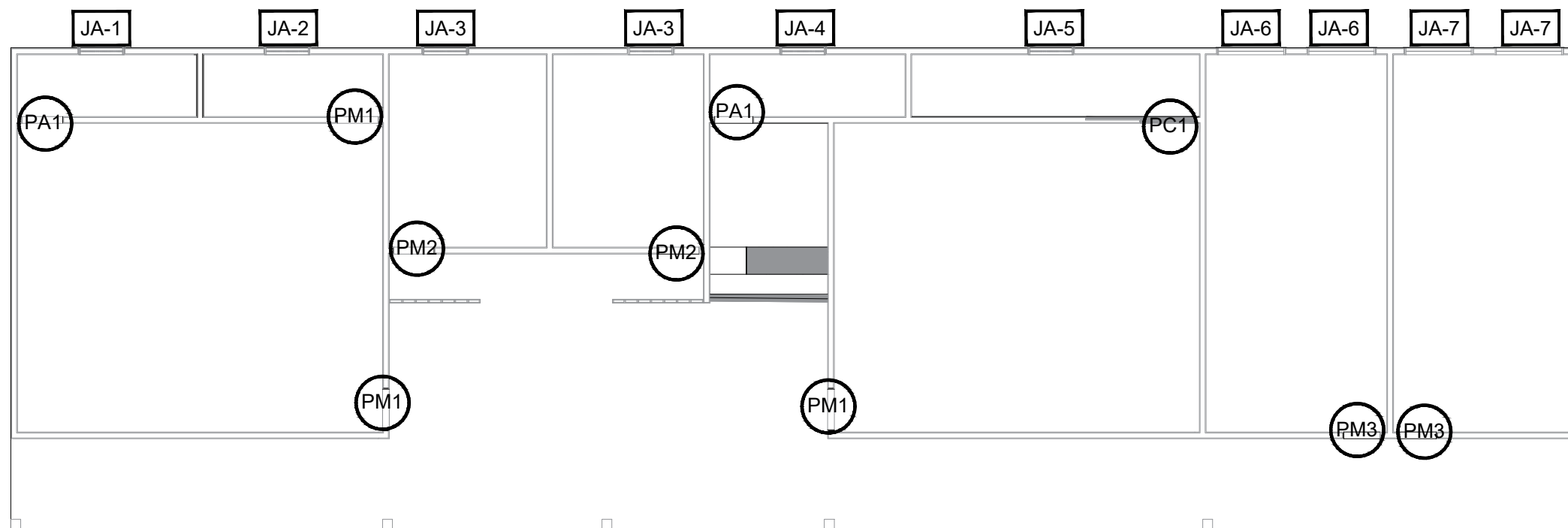
PLANTA BAIXA DETALHAMENTO DE ESQUADRIAS esc 1:125
